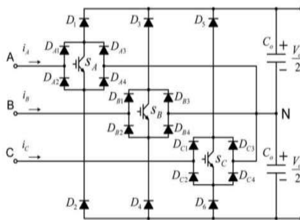
Fig: 1 Vienna Rectifier
