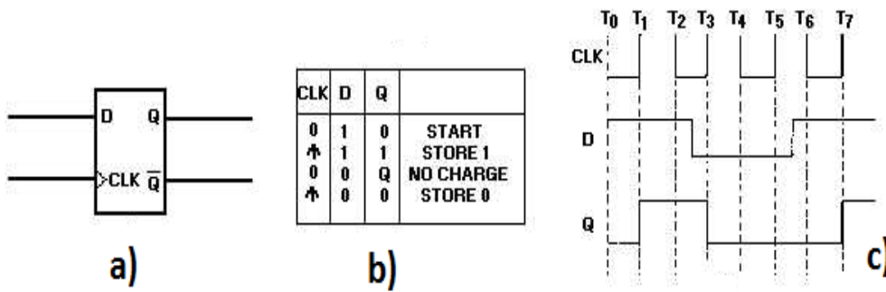
Fig. 6 a) D-FF standard symbol. b) Truth table c) Timing diagram
